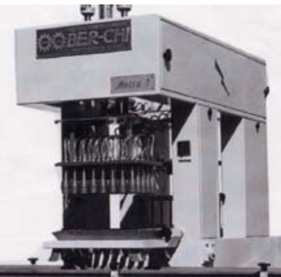
Incassettatrice per bottiglie, 1970
